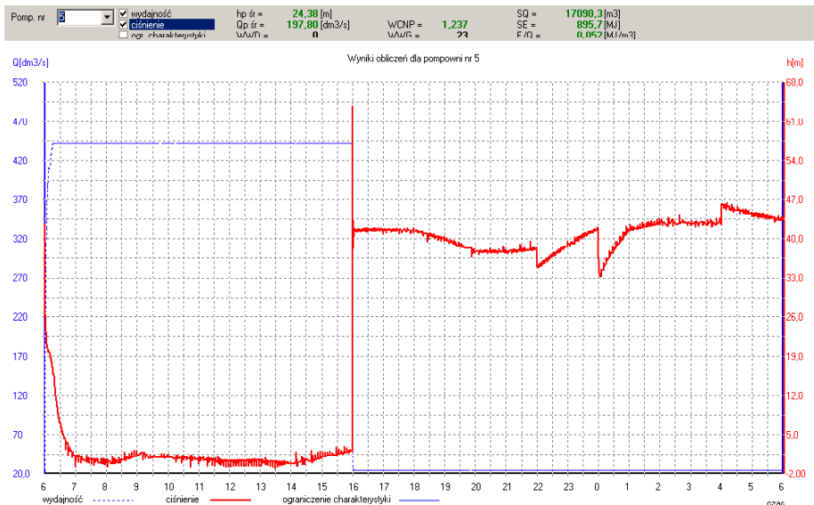
Rysunek 4.B5. Wykres czasowego przebiegu parametrów pracy pompy P5 w pompowni Jurowce (węzeł nr_23) dla wariantu B5
