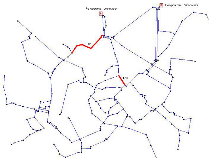
Rysunek 1.B. Schemat PDW Białegostoku z wyróżnionymi badanymi elementami wariantu B
